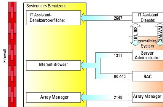
Abbildung 11-1. Typische Installation hinter einer Firewall
