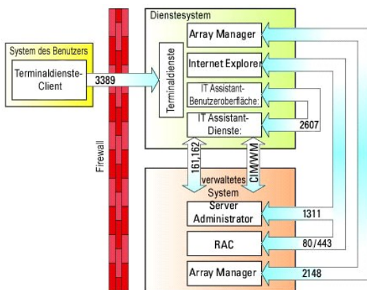
Abbildung 11-2. Terminaldienste für zusätzliche Sicherheit verwenden
